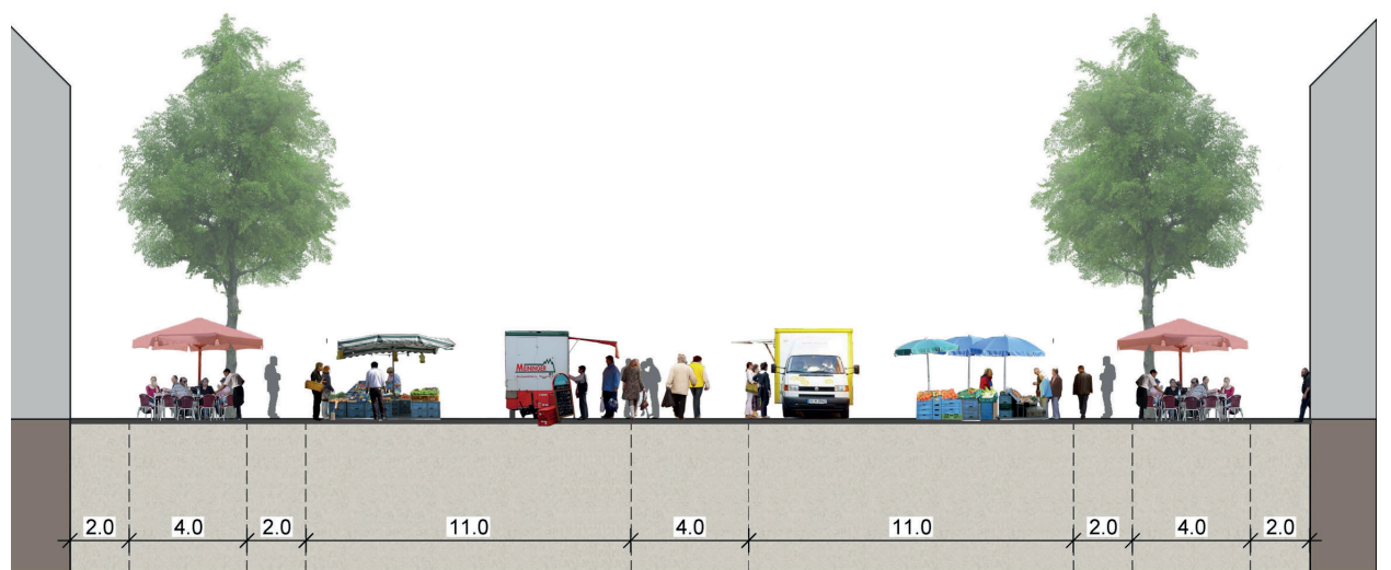
Systemschnitt Marktplatz
